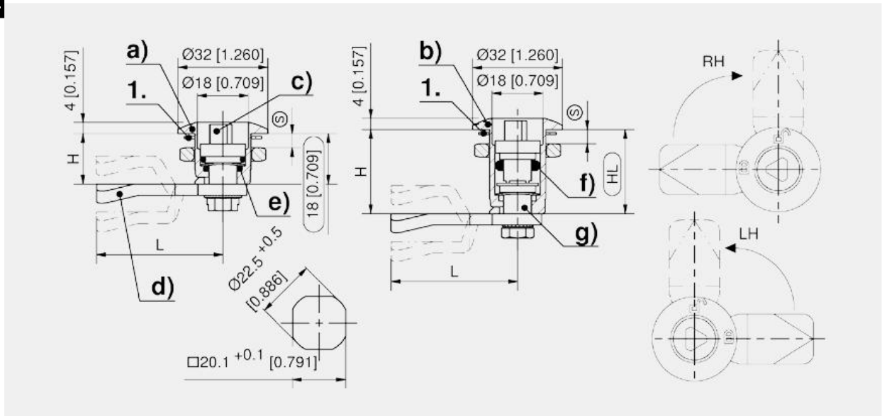
НКорпус с индикатором "открыто/закрыто", плоским уплотнением и заземляющей гайкой
