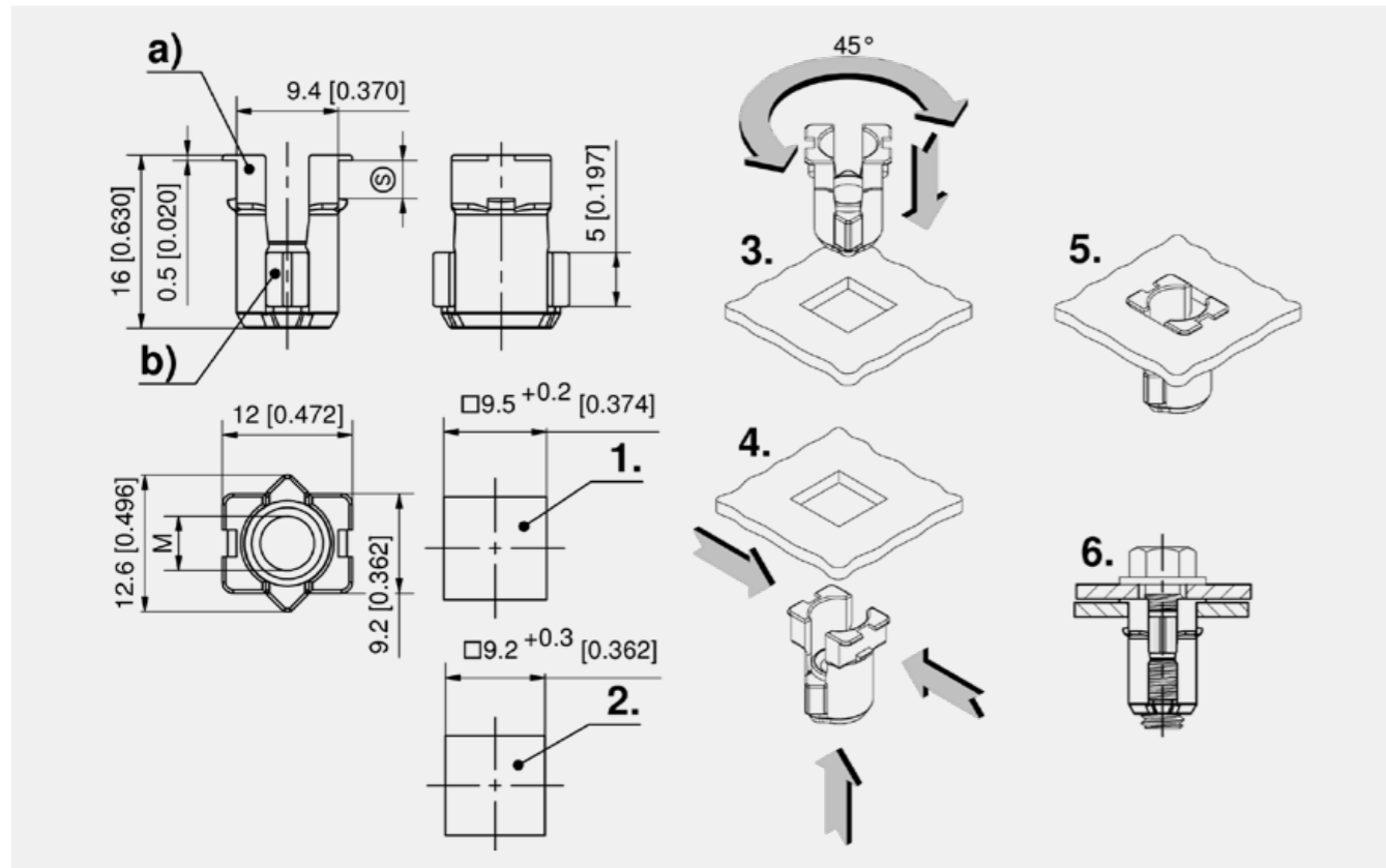
Закладная гайка, в разобранном виде
