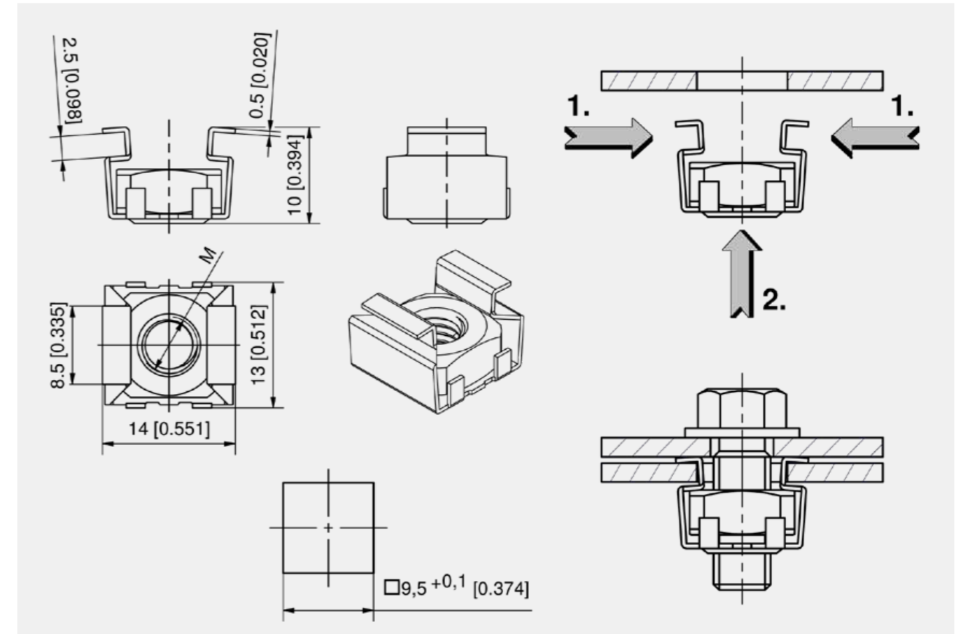
Закладная гайка
